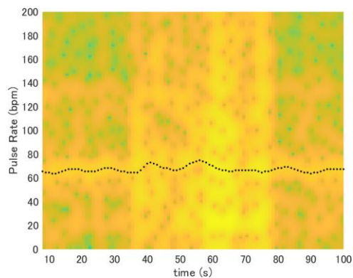
NIR光脈波の周波数スペクトル (黒線は正解脈拍数)
